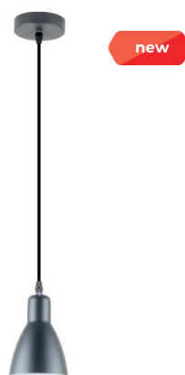
MORA | Pendant lamp A8102-1 1 x E27 MAX 40W Ø11 H141,5 metal black body, white shade inside
